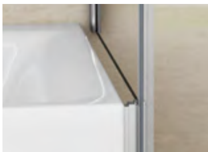
■ A rövidített oldalfal kádhoz való csatlakoztatásának részletei
