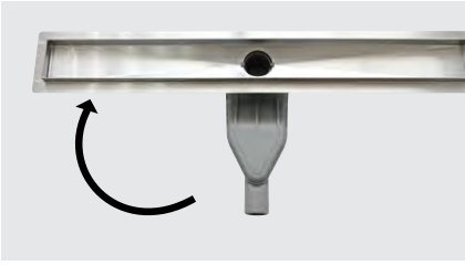
360 fokban forgatható szifon
