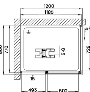
TRITON + TRITON BLACK ZUHANYKABIN
