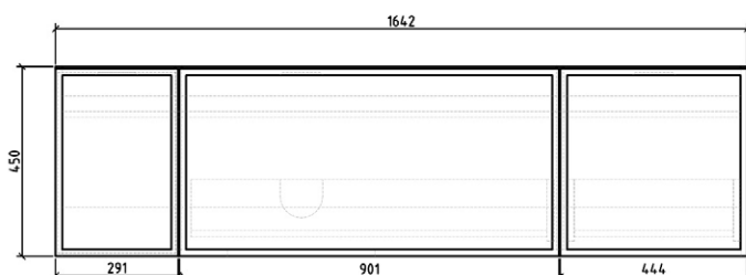
TRIPOLI MOSDÓSZEKRÉNY ÉS PORCELÁN TOP
