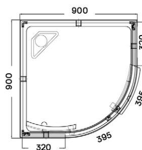
VIVARA HÁTFALAS ZUHANYKABIN TÁLCÁVAL
