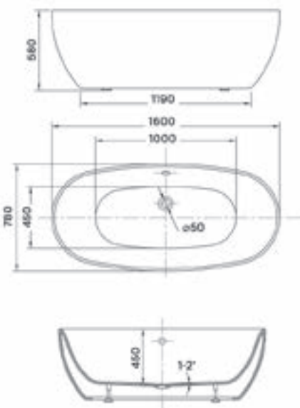
OVAL 160 SZABADON ÁLLÓ KÁD
