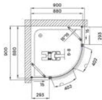
SCORPIO ZUHANYKABIN
